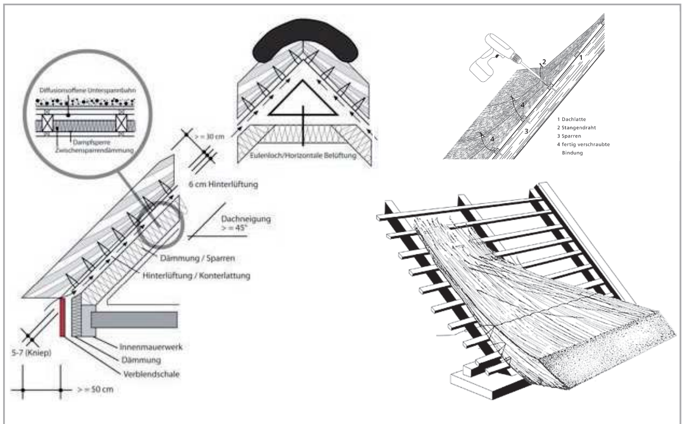
Abbildung 1: Aufbau eines Reetdaches [ http://www.baubegriffe.com , http://www.pro-reet.de ]
