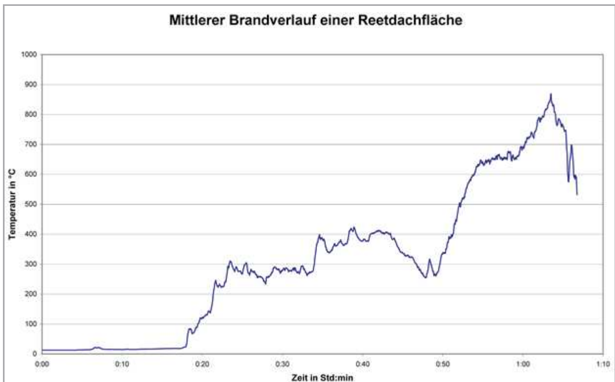
Abbildung 2: Temperaturverlauf Reetdach von Brandversuch der FH Lübeck
